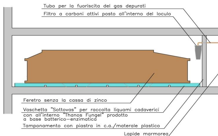
Schema loculo aerato - Immagine tratta da sito commerciale
